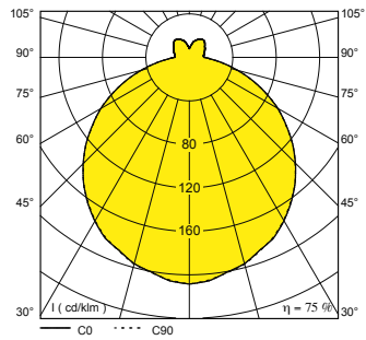
Lichtstärkeverteilung
